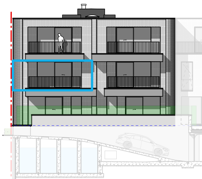
ACHTERGEVEL
