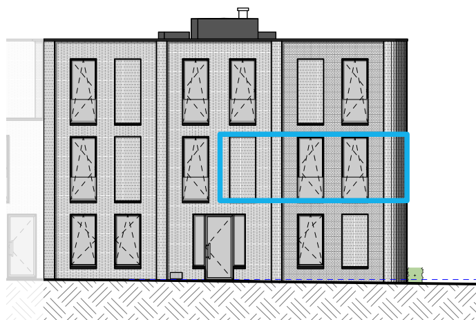
VOORGEVEL
